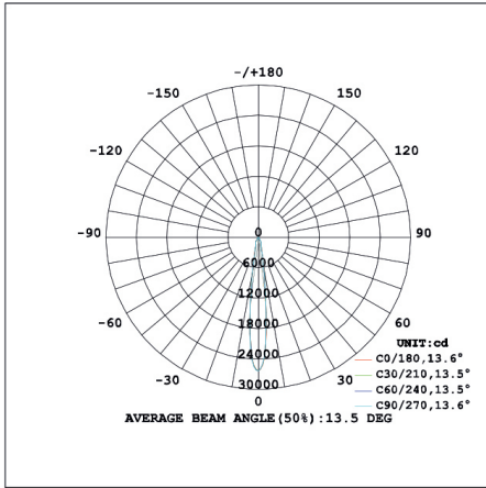
CRI80 15°
