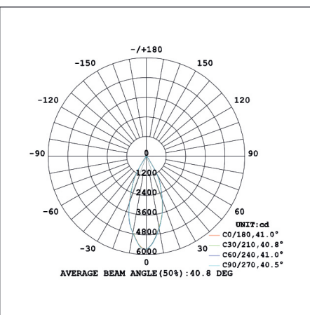
CRI80 45°
