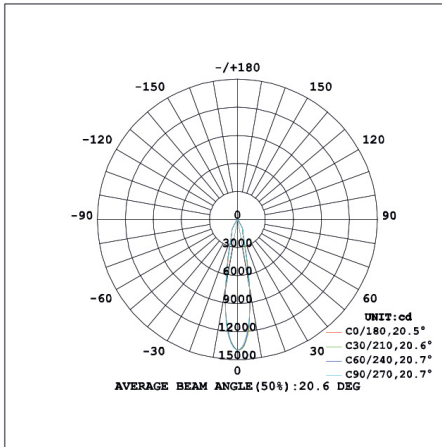
CRI80 20°
